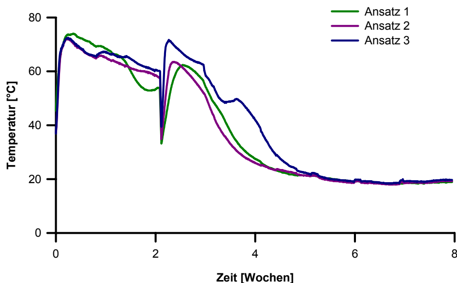
Abb. 3-1: Verlauf der Maximaltemperaturen in den Ansätzen A1, A2 und A3 während der Reaktorrotte
