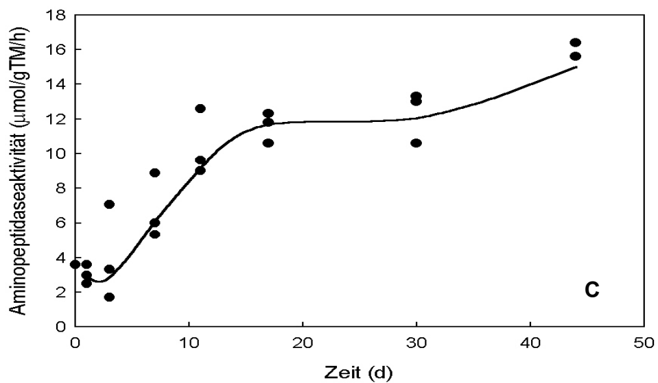
Abb. 7-1: Kompostierexperiment I: A: Mittlere Temperatur während der Kompostierung, B: Gesamtkeimzahl, C: Amino peptidaseaktivität
