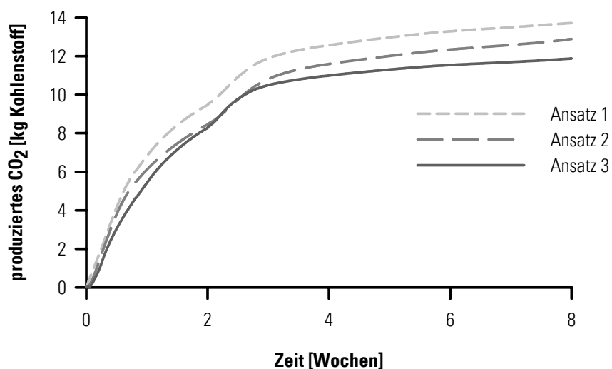
Abb. 5-1: Kohlenstoffdioxid-Produktion in den Ansätzen mit unterschiedlichem Störstoffgehalt (Ansatz 1: störstoffarm; Ansatz 2: Störstoffanteil 1 Mass.-%; Ansatz 3: Störstoffanteil 2,6 Mass.-%); die Kurvenverläufe wurden über die online-Messdaten integriert
