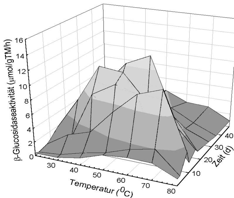
Abb. 7-6: Kompostierexperiment II: Dreidimensionale Darstellung der \beta -Glucosidaseaktivität in Abhängigkeit von Zeit und Temperatur während der Kompostierung
