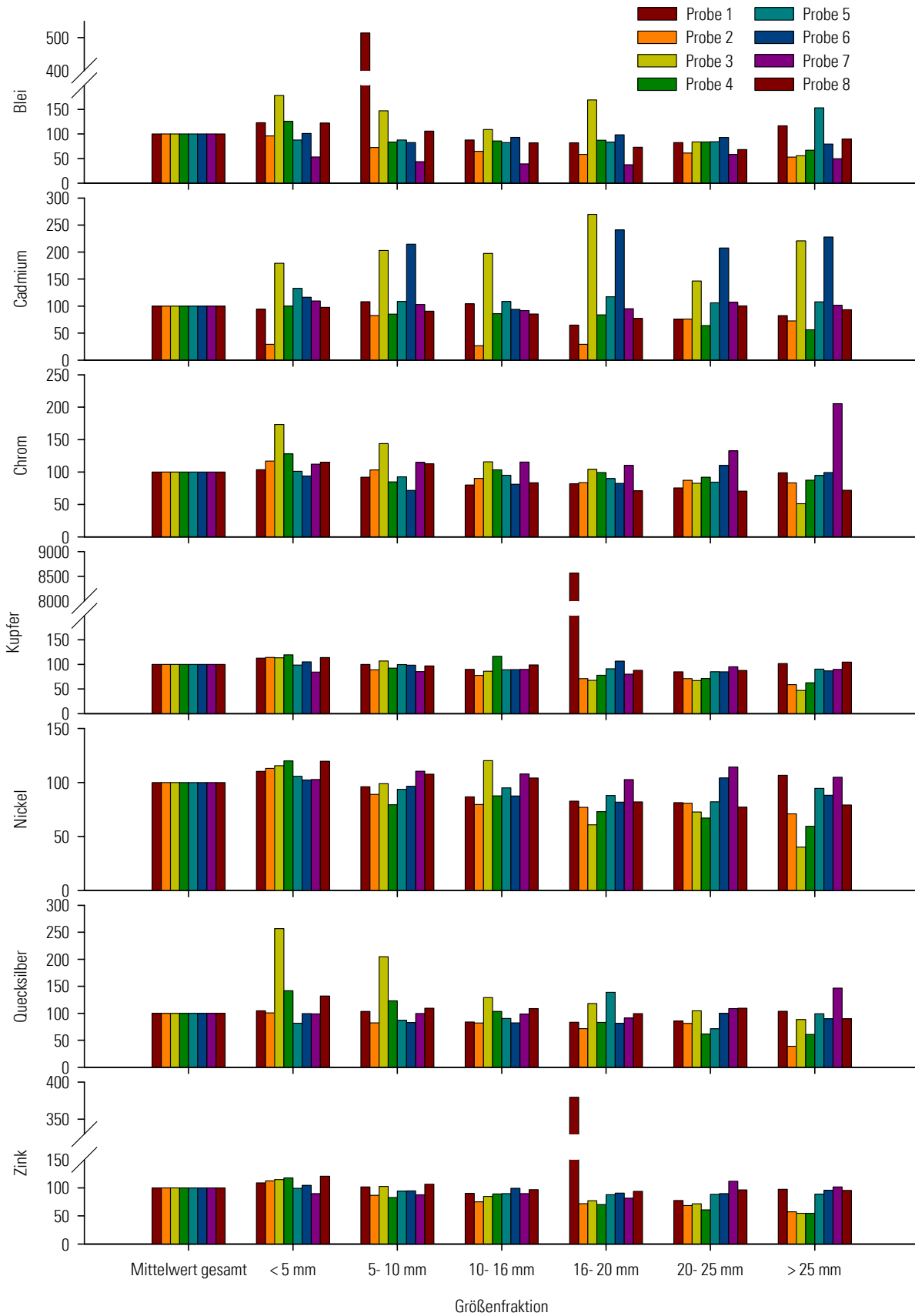
Abb. 6-1: Schwermetallgehalte der Größenfraktionen 1 – 6 der einzelnen Kompostproben; die Schwermetallgehalte der Größenfraktionen sind normiert auf den Schwermetallgehalt der jeweiligen unfraktionierten Gesamtprobe
