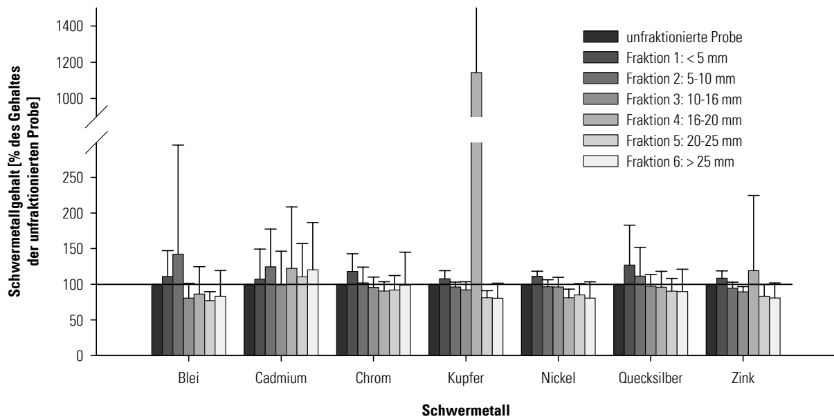
Abb. 6-2: Mittlere Schwermetallgehalte sowie Standardabweichung der sechs Größenfraktionen der Kompostproben; die Schwermetallgehalte der Größenfraktionen sind normiert auf den mittleren Schwermetallgehalte der unfraktionierten Gesamtproben
