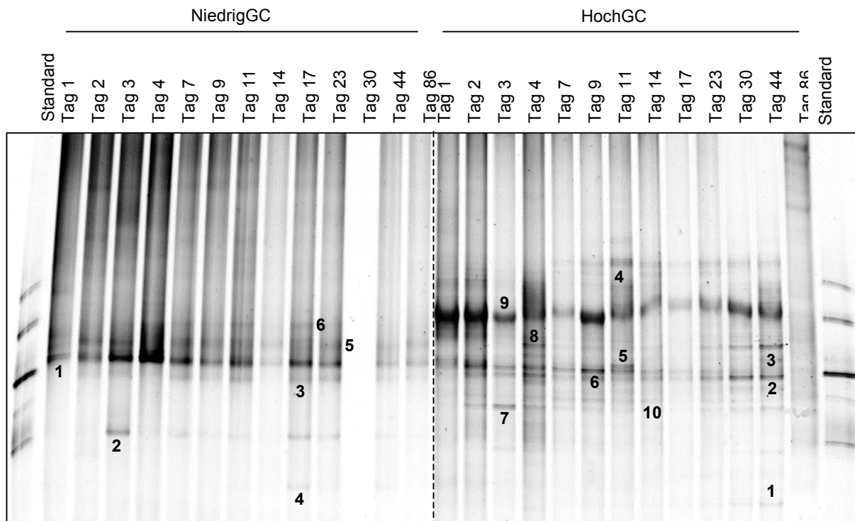
Abb. 7-4: Kompostierexperiment I: DGGE der PCR-Produkte von NiedrigGC- und HochGC-Gram-positiven Bakterien; die Ziffern symbolisieren die Schmelztypen
