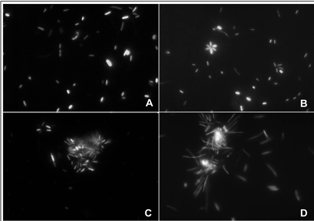
Abb. 7-2: Epifluoreszenzmikroskopische Aufnahme von Bakterien in Probenmaterial des ersten Kompostierungsversuchs; A: Tag 1; B: Tag 4; C: Tag 9; D: Tag 14
