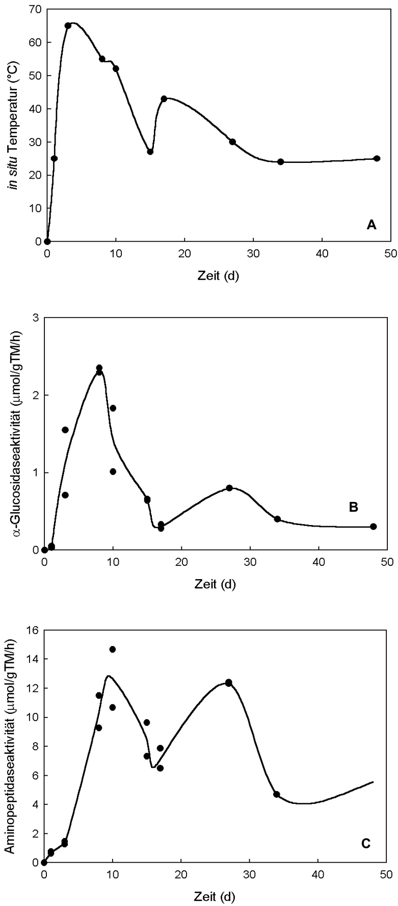
Abb. 7-5: Kompostierexperiment II: A: Mittlere Temperatur während des Kompostierversuchs; B: \alpha -Glucosidaseaktivität; C: Leucin-Aminopeptidaseaktivität
